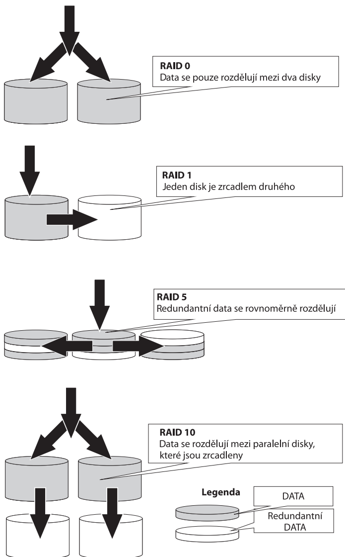
Obrázek 2.1: Princip RAID
