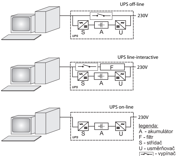
Obrázek 2.2: Principy UPS
