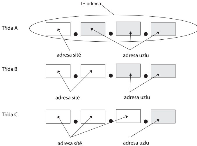
Obrázek 2.7: Třídy TCP/IP
