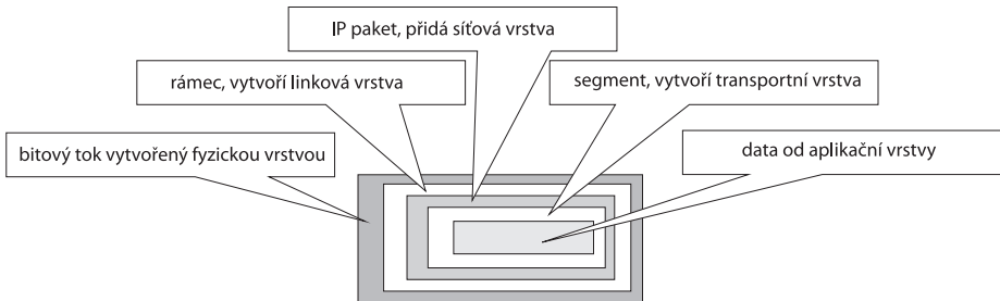
Obrázek 2.13: Zapouzdření
